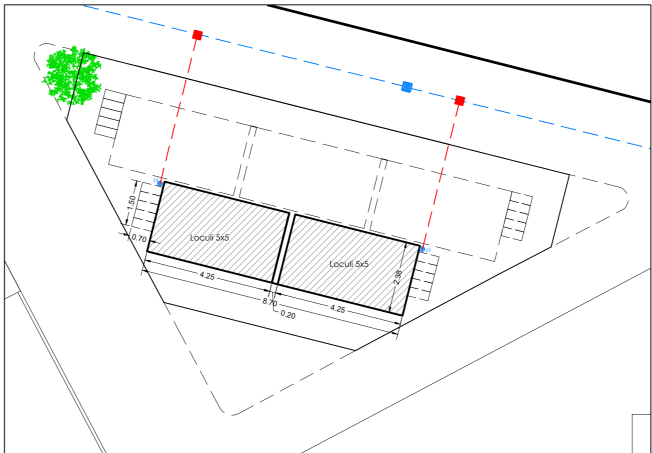
PLANIMETRIA GENERALE PROGETTO -scala 1:100-
